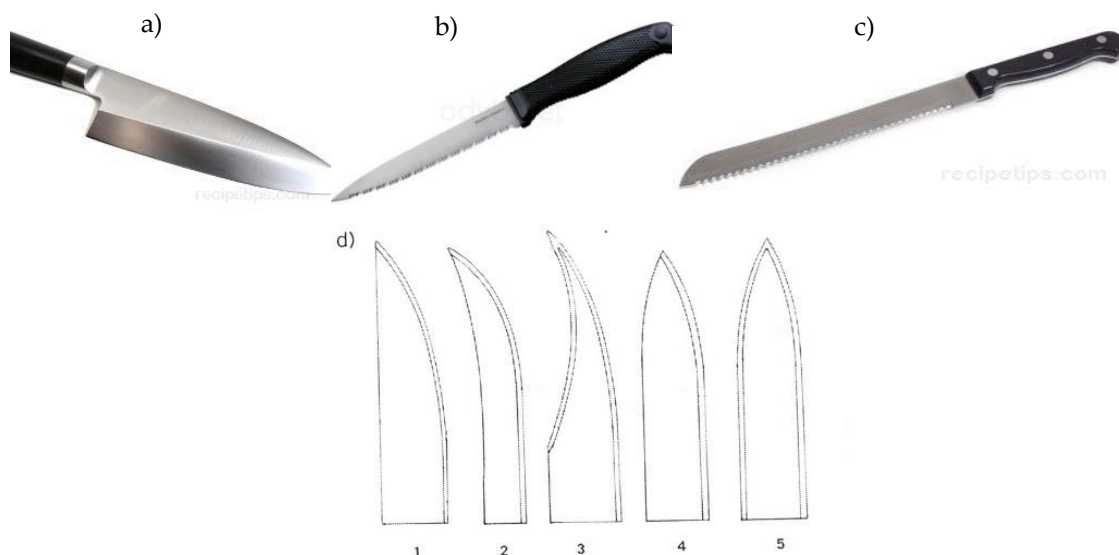
Расми 23. а) корди тезкунаки ҳамвор бо лаби буриши V-шакл; б) корд бо лаби буриши дандондор ва дандонҳои тез; с) корд бо лаби буриши аррадор ва дандонҳои доирашакл; д) шаклҳои тез
