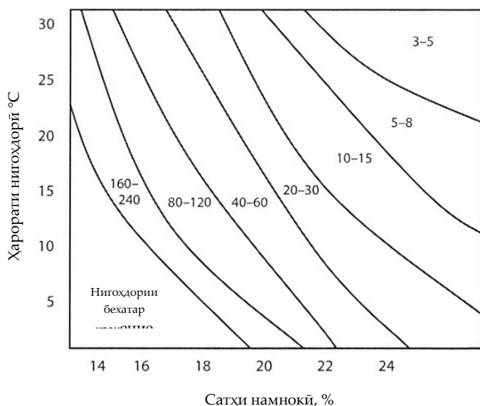
Расми 18. Таркиби бехатарии намӣ дар маҳсулот ҳангоми ҳарорати гуногуни нигоҳдорӣ
