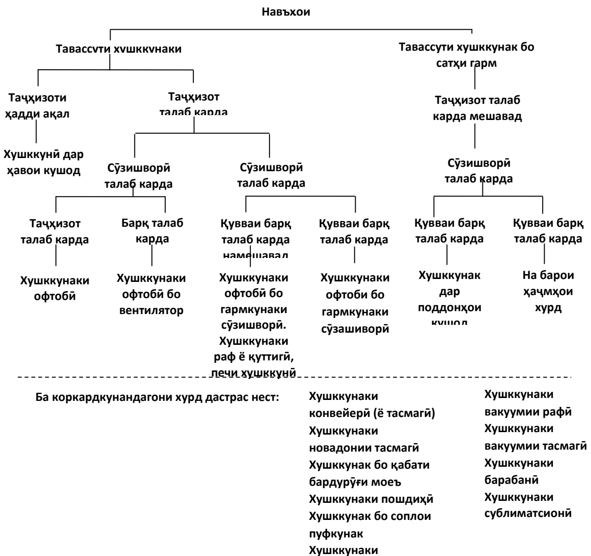
Рисунок 35. Типы сушилок
